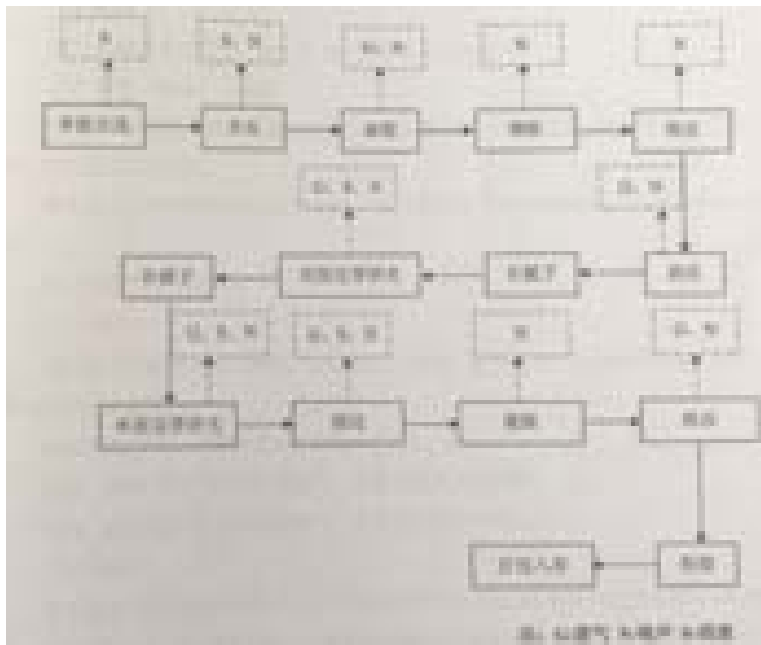
图 5.6-1 胶合板生产工艺流程图
